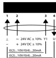
Электрическое подключение
