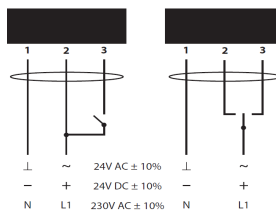
Электрическое подключение
